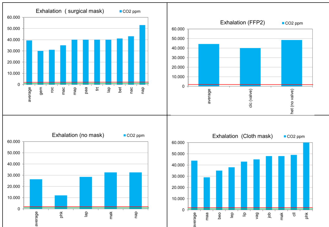
Figure 2. Grafici riassuntivi che mostrano i valori di CO 2 durante l' espirazione con i diversi tipi di mascherine
